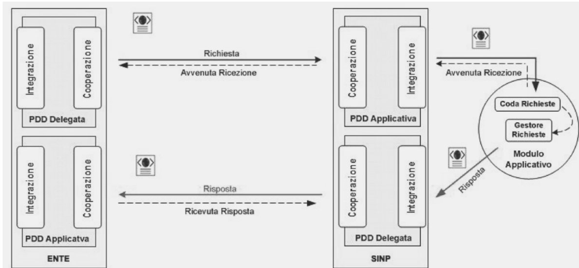
Figura 2 - Profilo Asincrono
